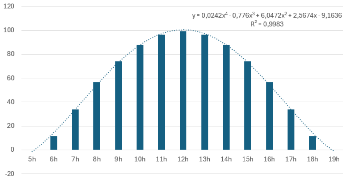
Fig.22 Energie produite par une surface élémentaire inclinée à 30° par rapport au plan horizontal lors du solstice d'été par 47°N
