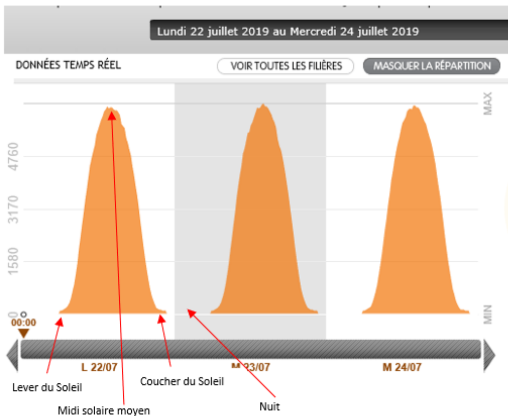
Fig.28 La production photovoltaïque s'apparente à un signal sinusoïdal mono-alternance.
