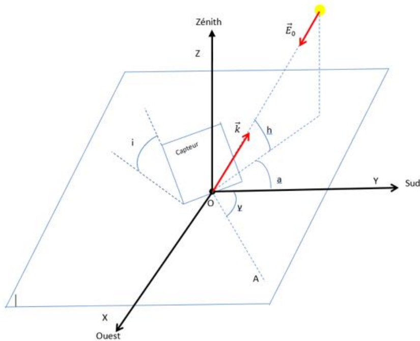
Fig.20 L'éclairement de la surface élémentaire dépend de son inclinaison i et de son azimut \gamma
