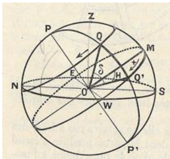
Fig.7 Les coordonnées horaires.
