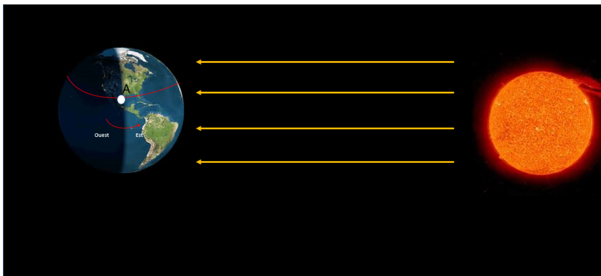
Fig.1 Le sens de rotation de la Terre. Un observateur qui est en A voit le Soleil dans la direction de l'Est. C'est le matin, la nuit vient de s'achever. La Terre tourne d'Ouest en Est, notre personnage passe de la nuit à la journée et observe le Lever du Soleil.
