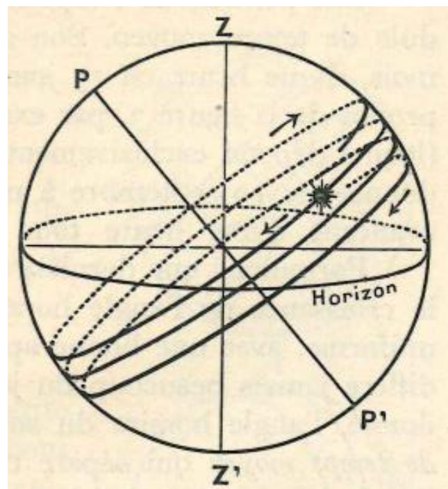
Fig.12 Mouvement apparent du Soleil sur la sphère céleste locale.
