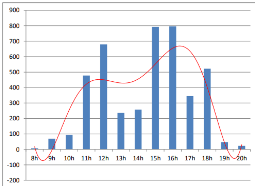
Fig.29 Eclairement solaire mesuré par le pyranomètre de l'observatoire météorologique de Saillé en Guérande le 31 mars 2018 par journée “ ciel variable ” En ordonnée le puissance mesurée, par unité de surface ( Wm^{-2} ). Nous sommes bien loin d'une demi-sinusoïde. (source : météociel)
