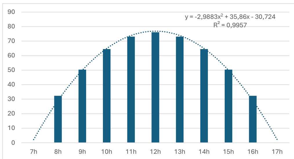
Fig.23 Energie produite par une surface élémentaire inclinée à 30° par rapport au plan horizontal lors du solstice d'hiver par 47°N
