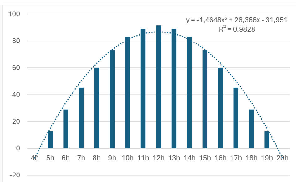
Fig.17 Eclairement d'une surface horizontale élémentaire au solstice d'été à une latitude de 47°N
