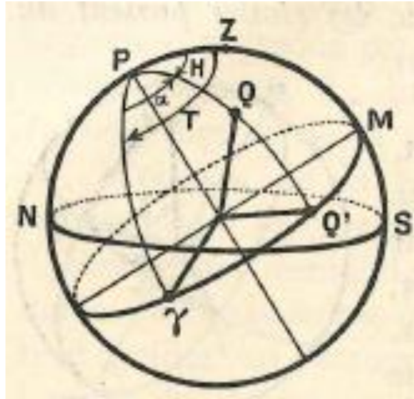
Fig.9 L'angle horaire du point \gamma à reçu un nom particulier on le nomme temps sidéral.
