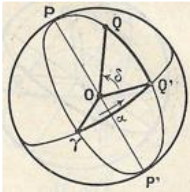
Fig.8 Coordonnées équatoriales.
