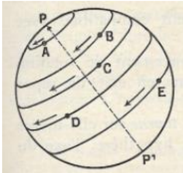
Fig.4 La sphère des fixes
