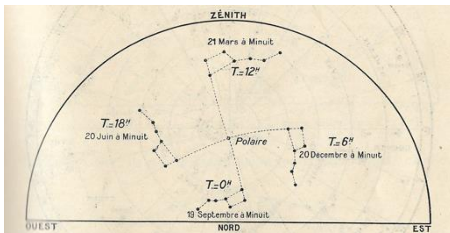
Fig.10 Position de la Grande Ourse dans le ciel, à diverses époques de l'année, à minuit, lorsque le temps sidéral est T=0h ; 6h , etc...
