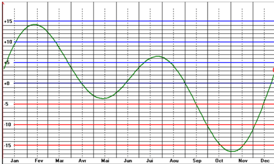
Fig.27 Le graphe représentatif de l'équation du temps. Il est suffisant pour la plupart des applications pratiques relevant de la physique appliquée.
