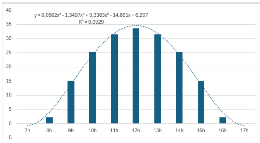
Fig.18 Eclairement d'une surface horizontale élémentaire au solstice d'hiver à une latitude de 47°N
