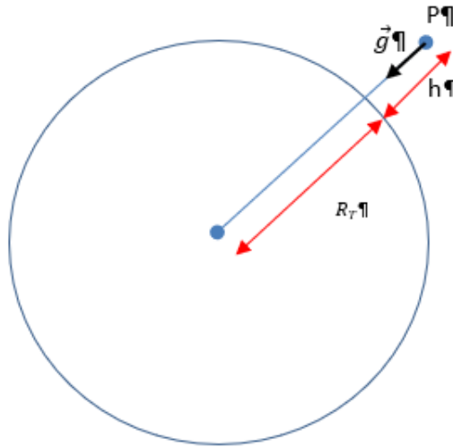
Fig.5. Le champ de pesanteur d'un astre varie en fonction de l'altitude
