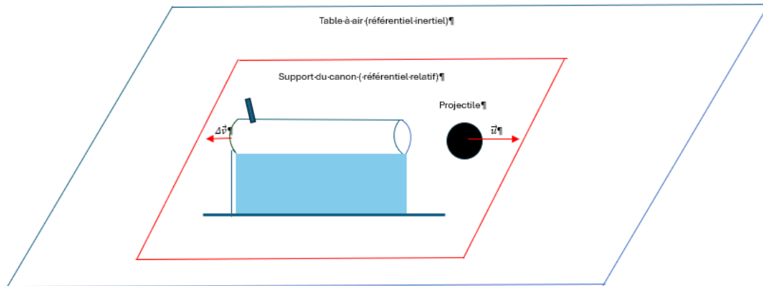
Fig.2. Indication du sens des vitesses après l'explosion.
