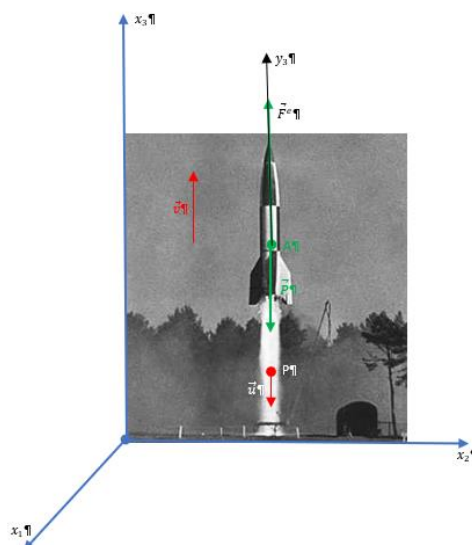
Fig.4. Le référentiel inertiel, terrestre ici, est représenté par le système d'axes (x_1, x_2, x_3) .
