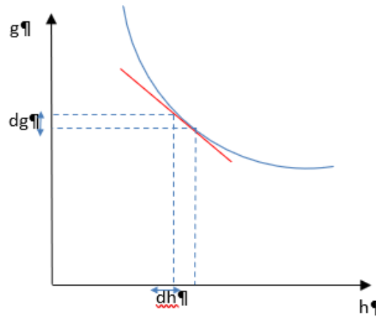
Fig.6. La formule (12 4 ) est une approximation linéaire de la variation du champ de pesanteur avec l'altitude.
